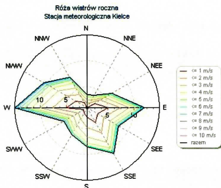
Rys. 1 Róża wiatrów dla Regionu Kieleckiego
