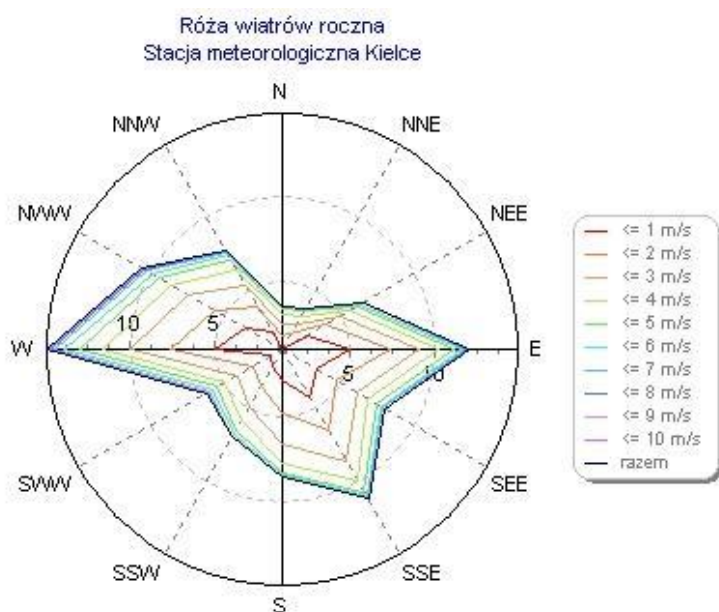
Róża wiatrów dla Regionu Kieleckiego
